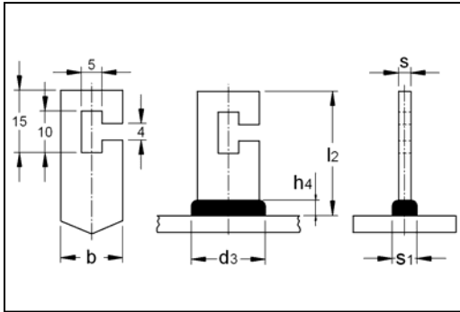
KÖCO KFS/C Flachstift Form C Rectangular stud type C Goujon rectangulaire C Espárrago rectangular C
